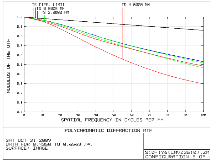
Iris dia. \phi 8.8 F1.9 Middle (f=6.0mm)
