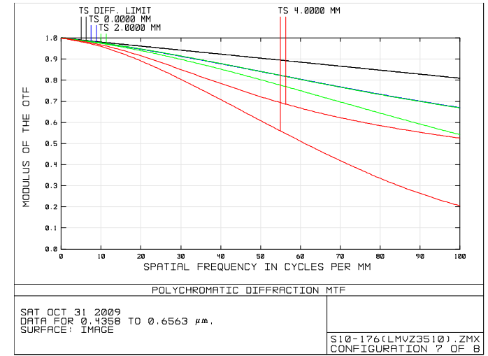
Iris dia. \phi 8.8 F2.6 Tele (f=9.8mm)
