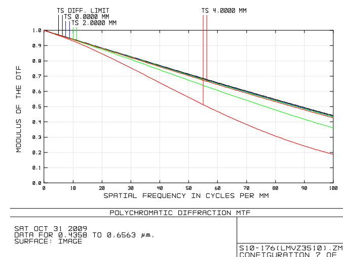
Iris dia. \phi 1.6 F11.0 Tele (f=9.8mm)
